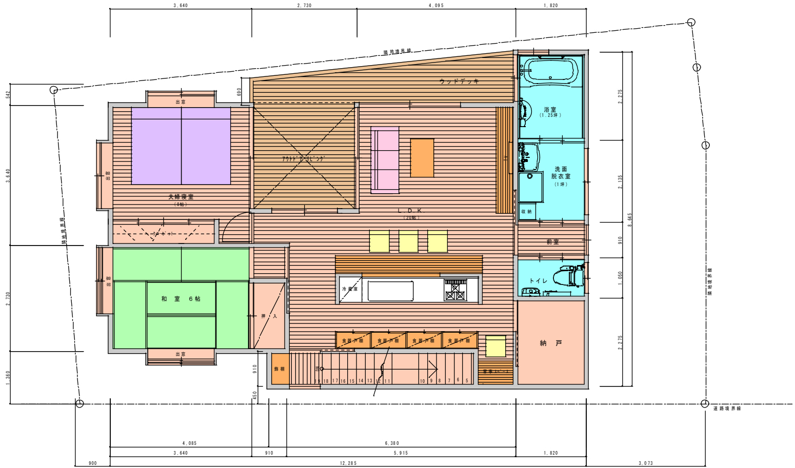
2階平面図 S=1/50
